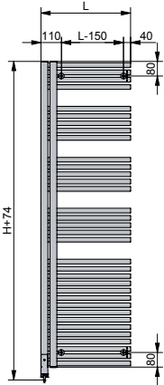
TLNSL - VUE ARRIÈRE
