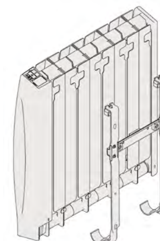
Vue arrière + Fixations :
