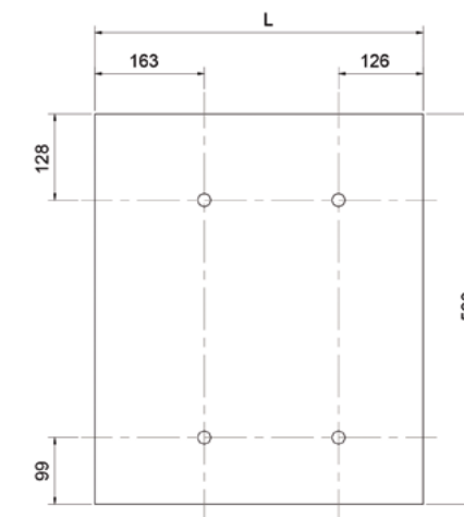
Repères de perçage :
