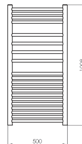
Vue de face 460 W :
