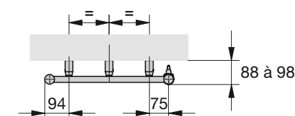
Saillie au mur : 88 à 98 mm
