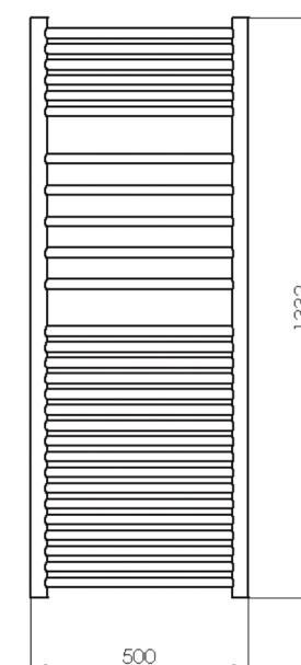
Vue de face 615 W :
