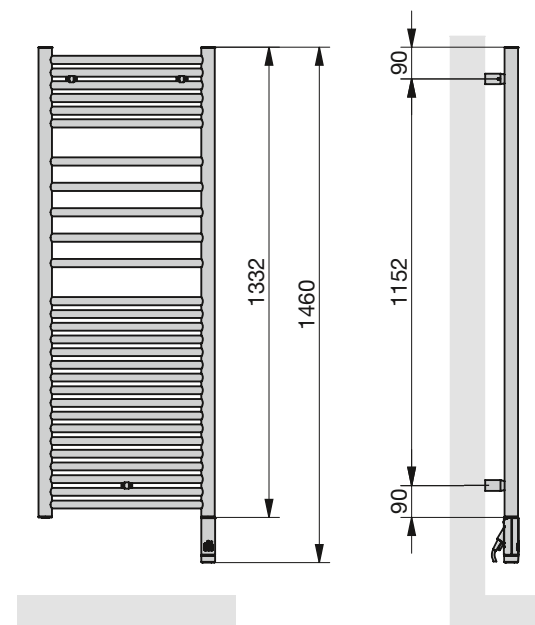
Vue de face 750 W :
