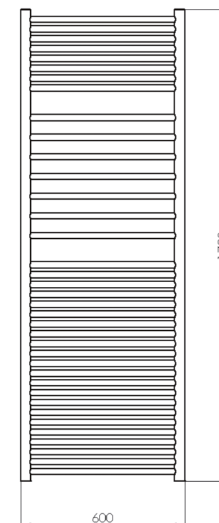
Vue de face 946 W :
